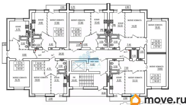
Блок секция А. План 2-10 этаж
