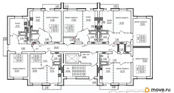
Блок секция А. План 2-10 этаж
