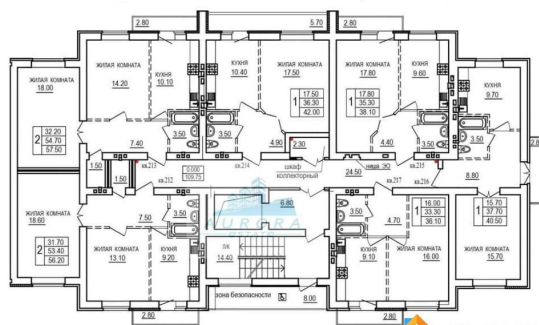
Блок секция Д, План 2-10 этажа
