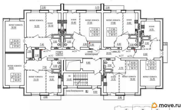
Блок секция Д. План 2-10 этажа
