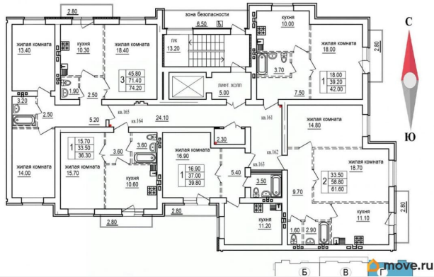
Блок секция Г. План 2-10 этажа
