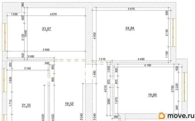
План обмерочный S=120\text{ м}^2
