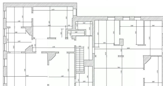
План 1 этажа
